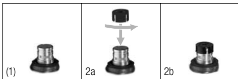
Fig. 4: Cápsula sin (1) y con (2b) el PB 1000
