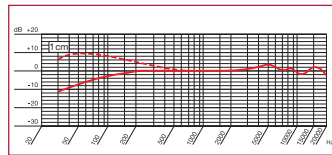
Abb. oben: Niere Abb. unten: Hyperniere (inklusive PPC 1000)
