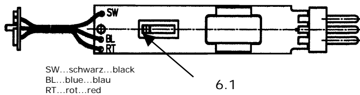
Verdrahtung zur Kapsel (M1:1) - Ansicht Bauteilseite wiring to capsule (Scale 1:1) - view comp.side
