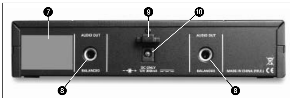
Fig. 2: Elementos de comando no painel de trás do receptor SR 40 DUAL
